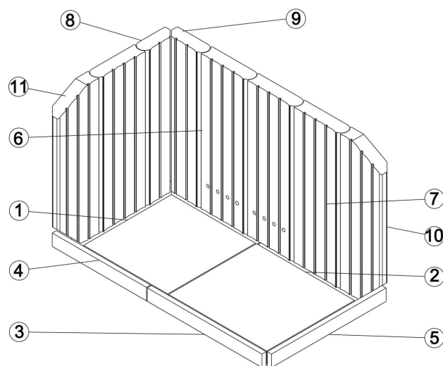
Abb. 1: Zusammenstellung der Schamottesteine Eck-Kamin 45/82/48 STR
